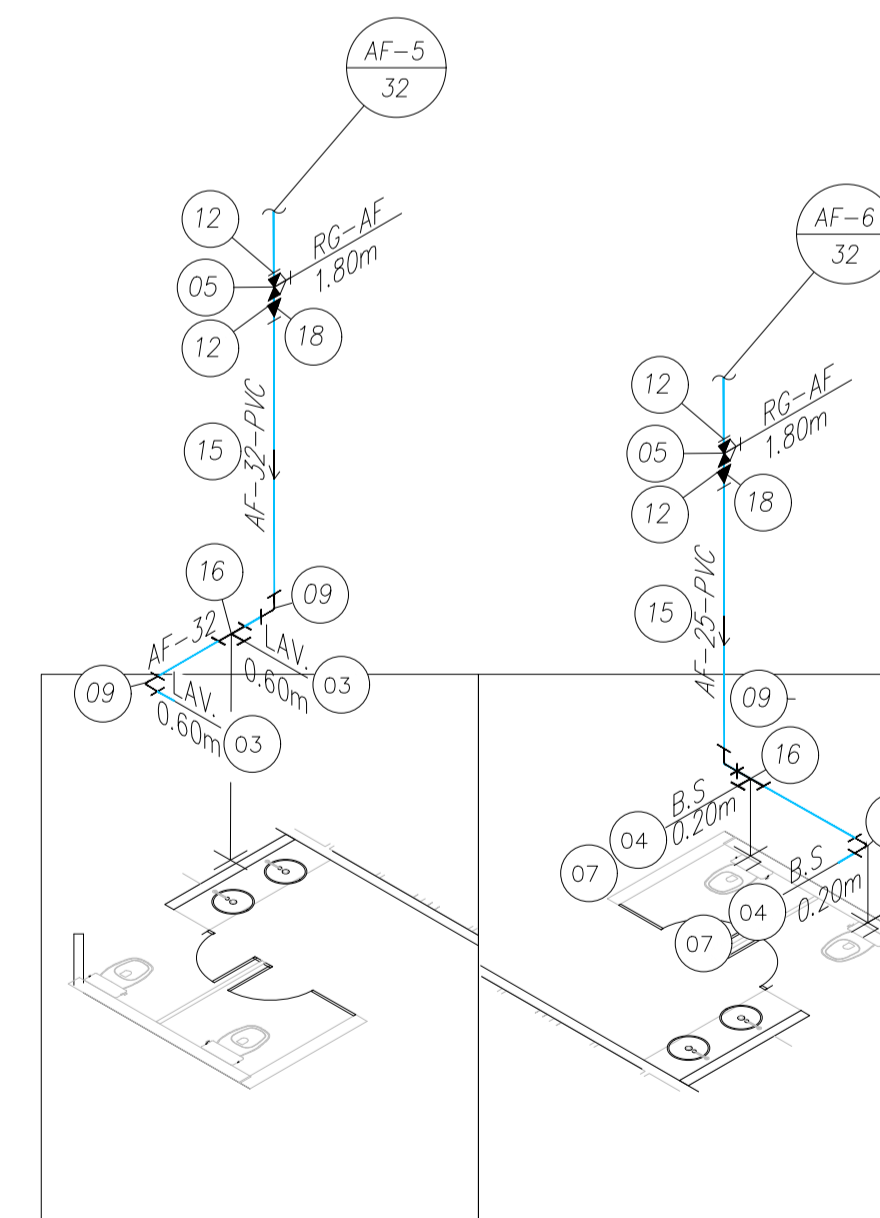
ISOMÉTRICO 08 33º PAVIMENTO ESCALA 1:25
