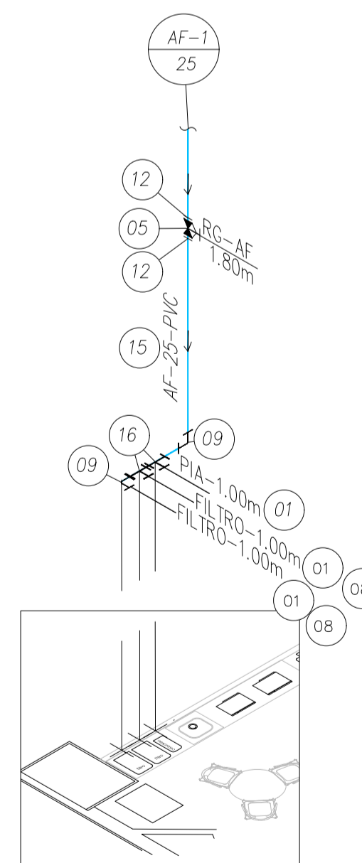
ISOMÉTRICO 05 33º PAVIMENTO ESCALA 1:25
