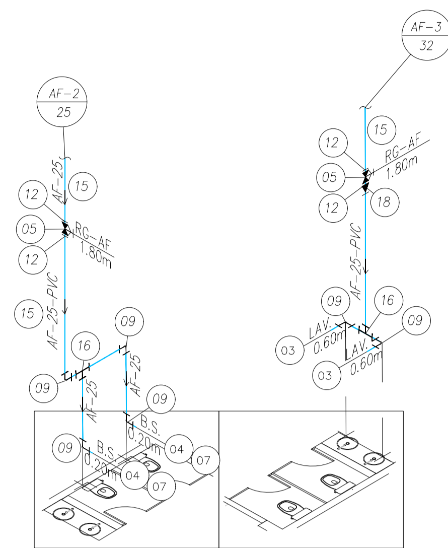
ISOMÉTRICO 02 32º PAVIMENTO ESCALA 1:25
