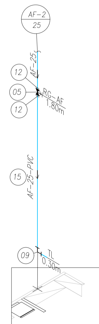
ISOMÉTRICO 06 33º PAVIMENTO ESCALA 1:25
