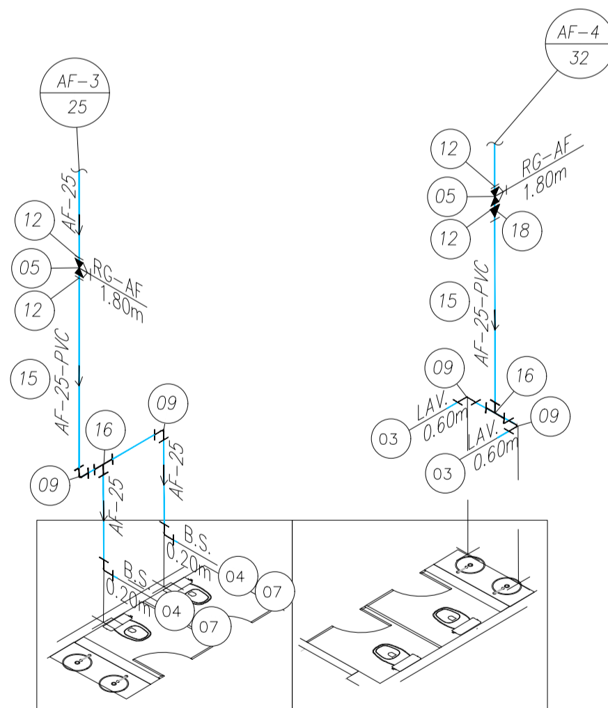
ISOMÉTRICO 07 33º PAVIMENTO ESCALA 1:25
