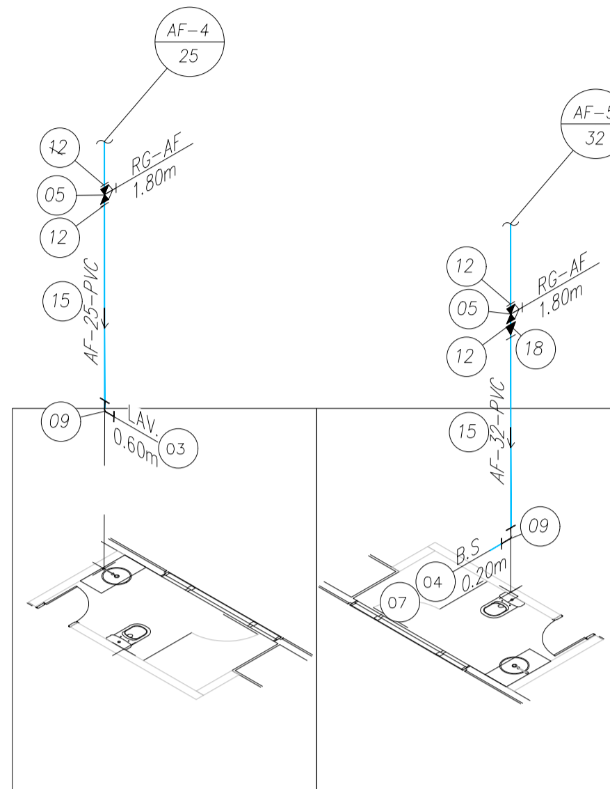
ISOMÉTRICO 03 32º PAVIMENTO ESCALA 1:25
