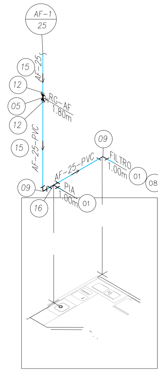
ISOMÉTRICO 01 32º PAVIMENTO ESCALA 1:25
