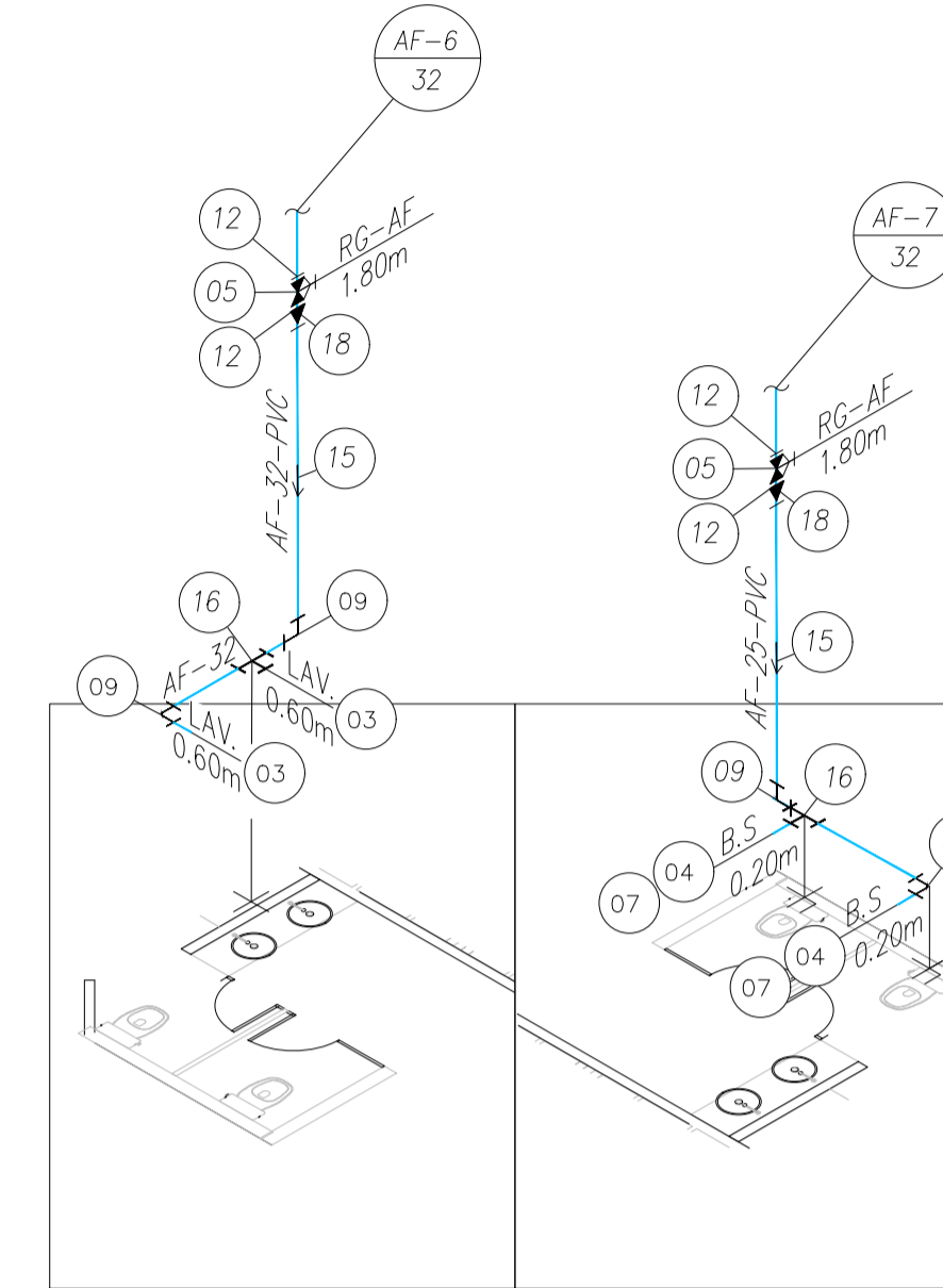
ISOMÉTRICO 04 32º PAVIMENTO ESCALA 1:25
