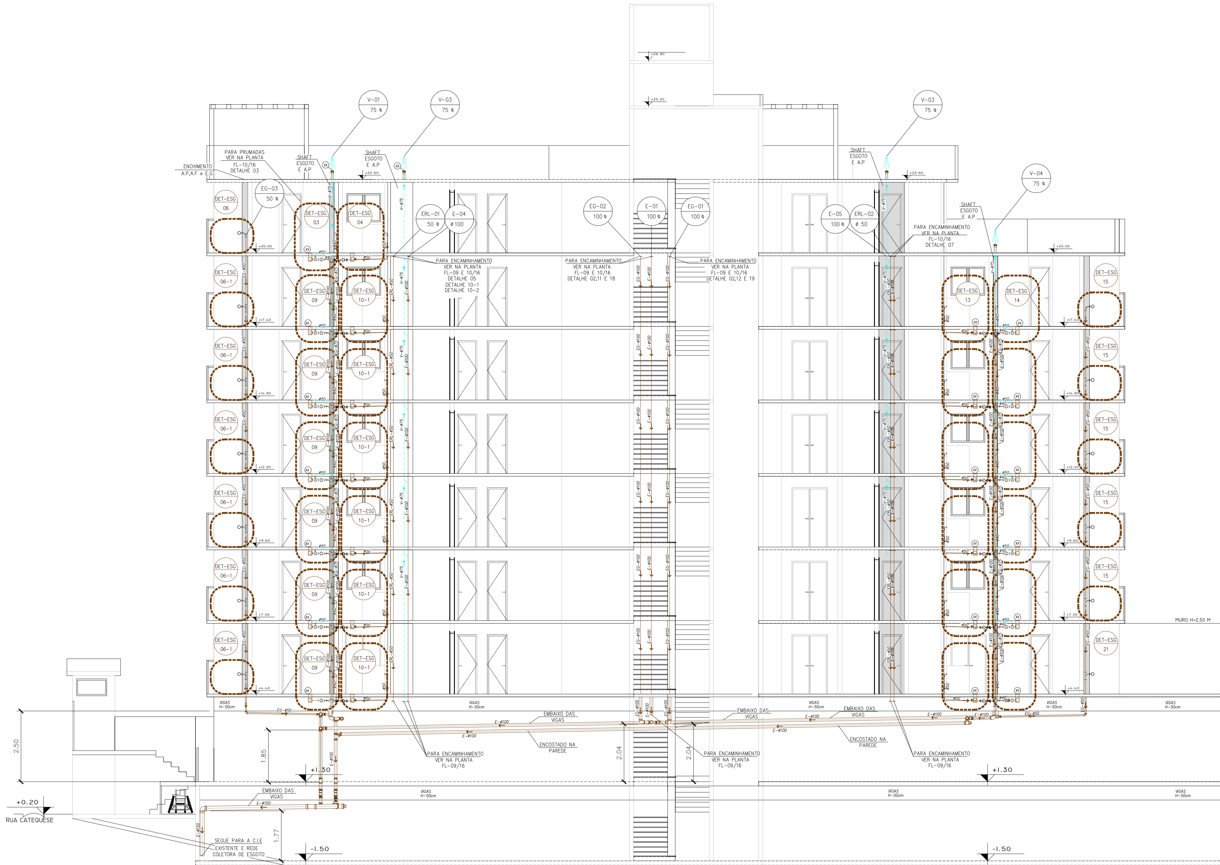
CORTE A.A PERFIL LONGITUDINAL
